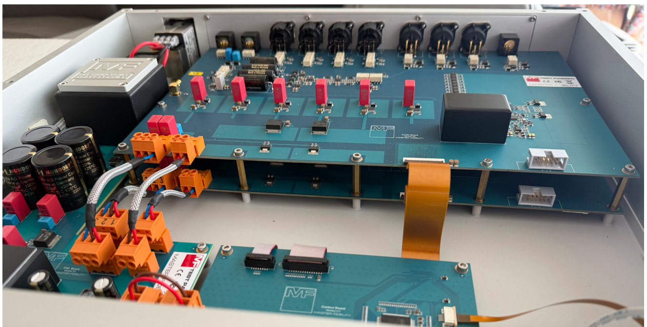
Duidelijke scheiding: besturing, voeding en analoge signaalverwerking zijn in de NADAC L strikt van elkaar gescheiden.
